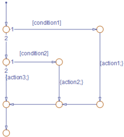
if-elseif-else
