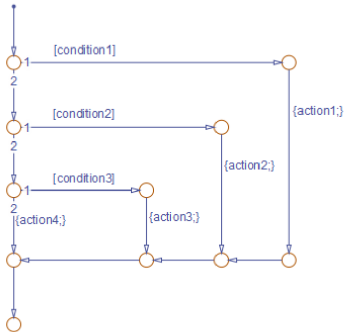
if-elseif-elseif-else
